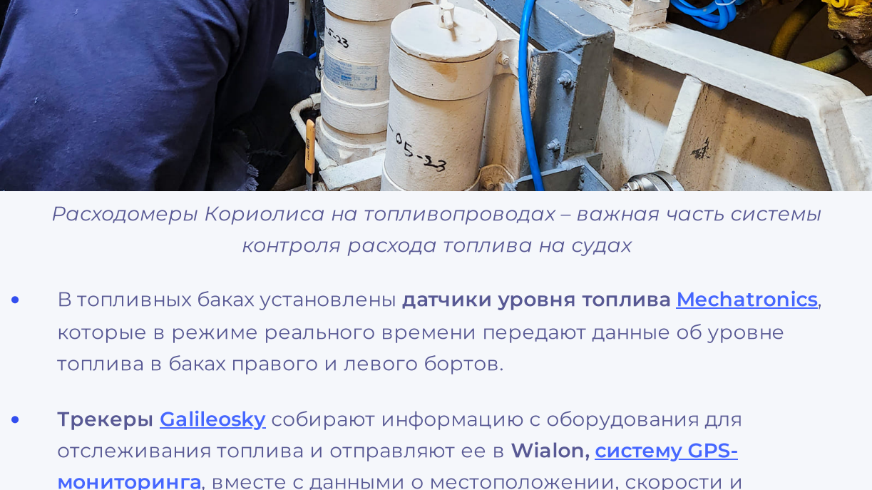
Расходомеры Кориолиса на топливопроводах – важная часть системы контроля расхода топлива на судах
